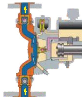
Чертеж поперечного сечения (*другие модели могут иметь иное строение)
