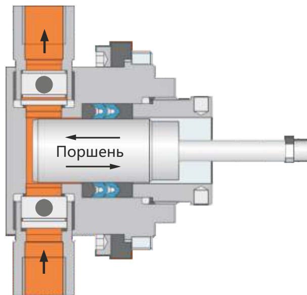
Чертеж поперечного сечения проточной части
